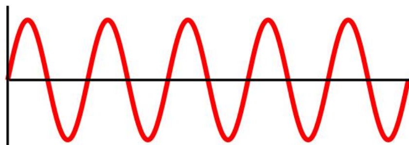
Constructieve interferentie
